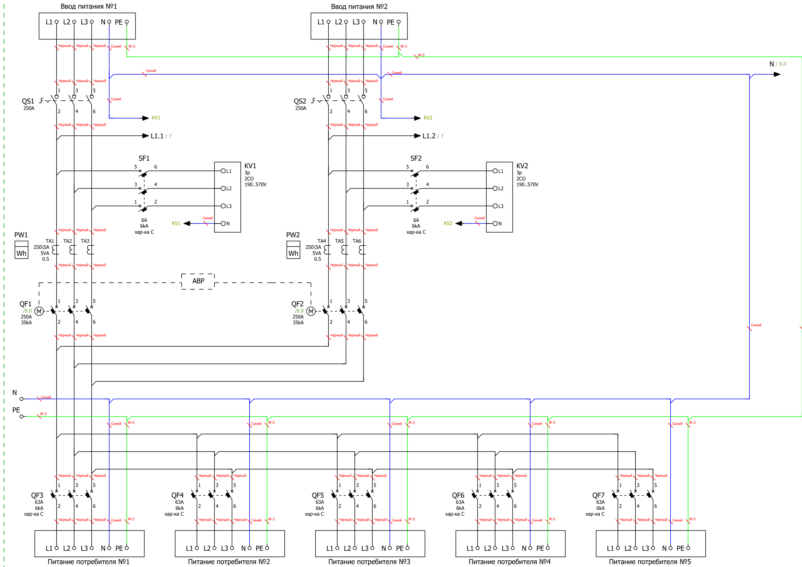
Схема электрическая силовая
